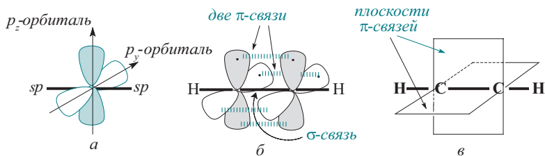
Рис. 1.8. sp -Гибридный атом углерода (а), схематичное изображение \pi -связей (б) и плоскостей \pi -связей (в) в молекуле ацетилена (гибридные орбитали показаны только осями)
