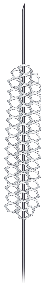
Рис. 3.6. Сетка
